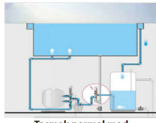
Taşmalı normal mod
