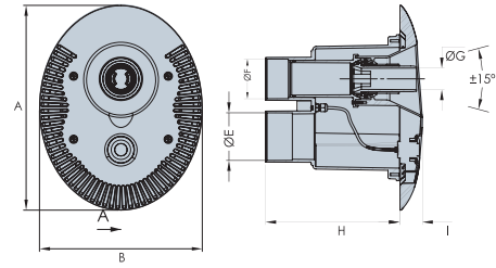
SECCIÓN A-A
